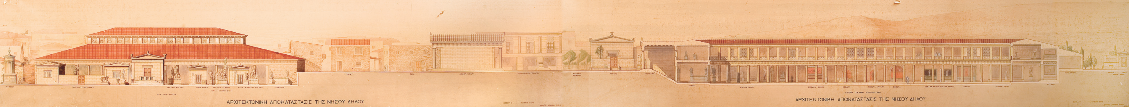
Alzados de la Sala Hipóstila y el Ágora de los Italianos de la ciudad de Delos. Jose Ignacio Hervada, 1937. RAER
