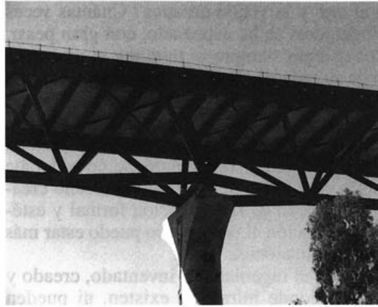
Figura 3.—Puede de García Sola (Badajoz, J. Manteola)
